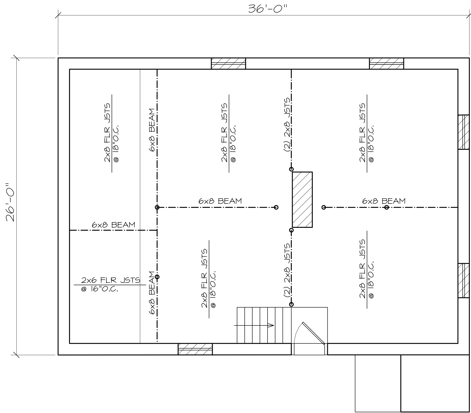
1 FOUNDATION PLAN A5 SCALE: 1/4" = 1'-0"
